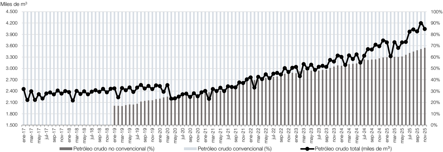
Gráfico 6.1 Extracción de petróleo crudo convencional y no convencional, en miles de m³ y estructura porcentual. Enero 2017-noviembre 2025
