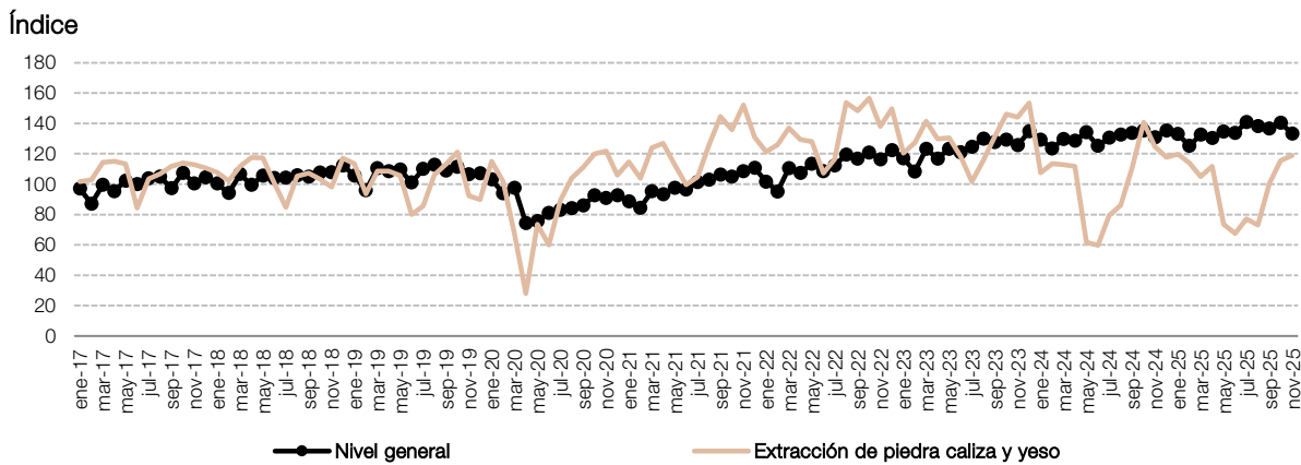
Gráfico 4.2.1 Extracción de piedra caliza y yeso respecto al nivel general del IPI minero, en números índice. Enero 2017-noviembre 2025
