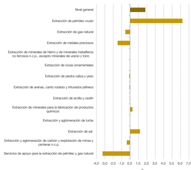
Gráfico 5.2 IPI minero nivel general y subclases, incidencias. Noviembre de 2025
